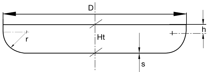
Fond plat avec grand rayon
