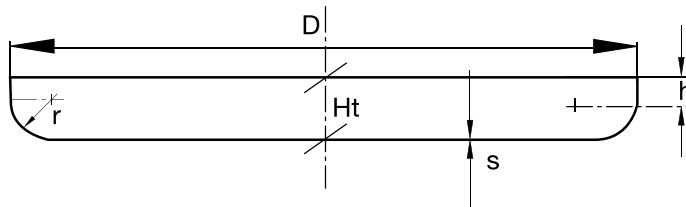
Fond plat avec petit rayon (p. 23)
