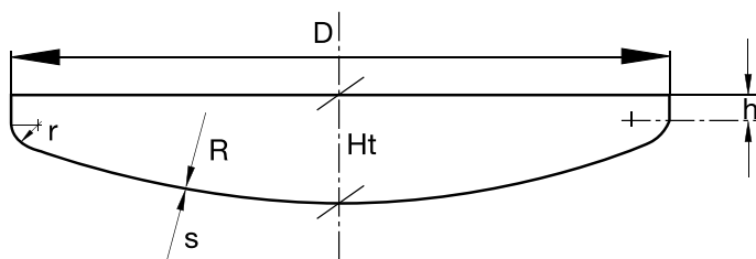
Fonds bombés a petit rayon de carre (p. 16-17)
