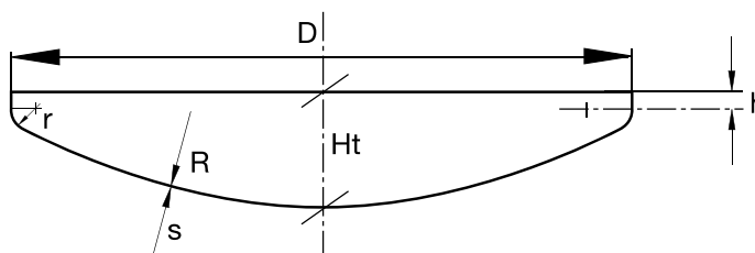
Fonds bombés a moyen rayon de carre (mrc) (p. 22)
